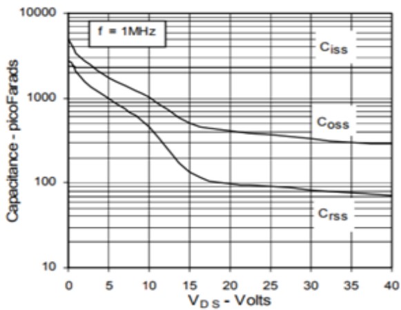
Fig. 11. Capacitance
